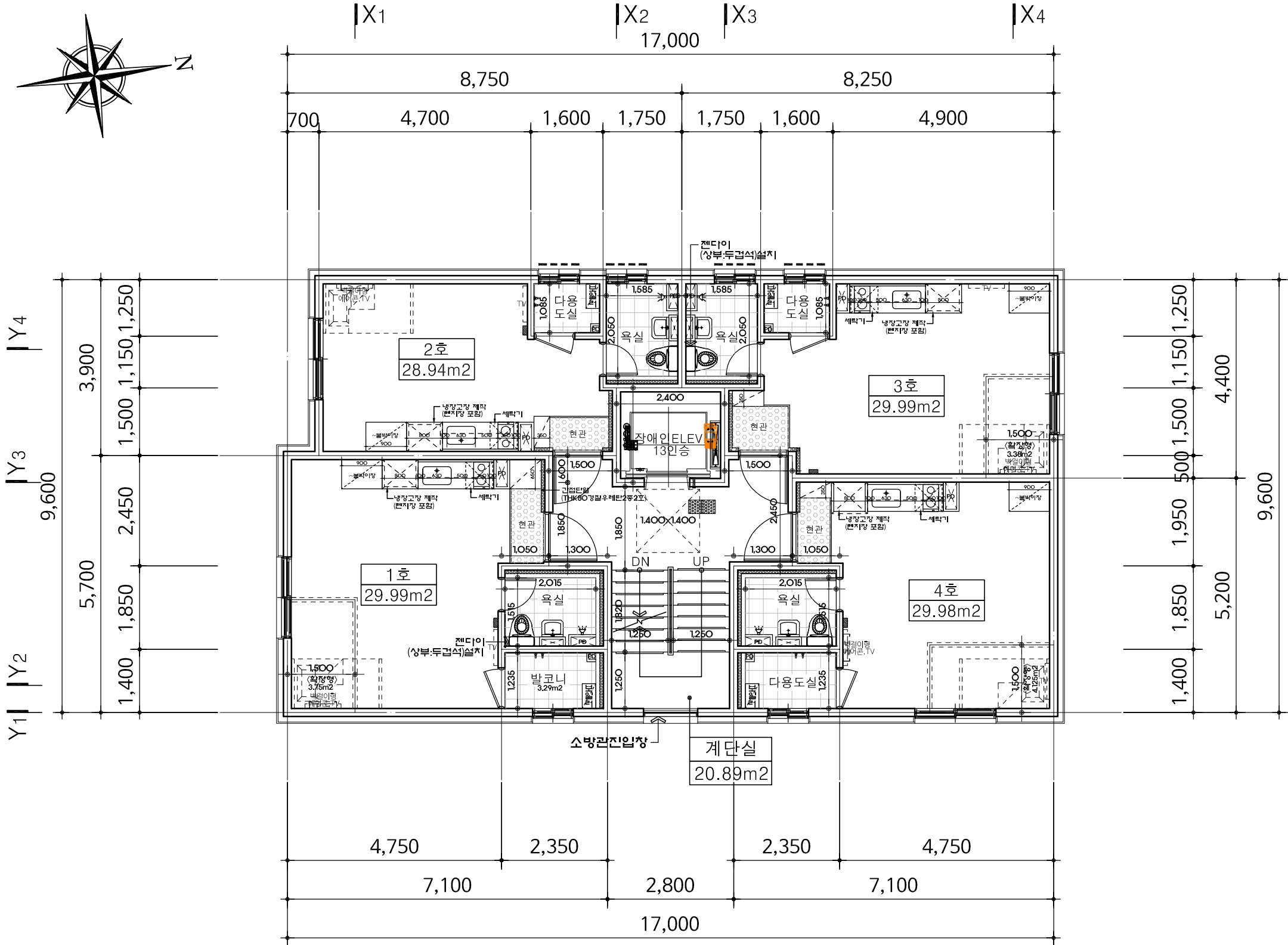
지상2~3층 평면도 축척: 1/100
