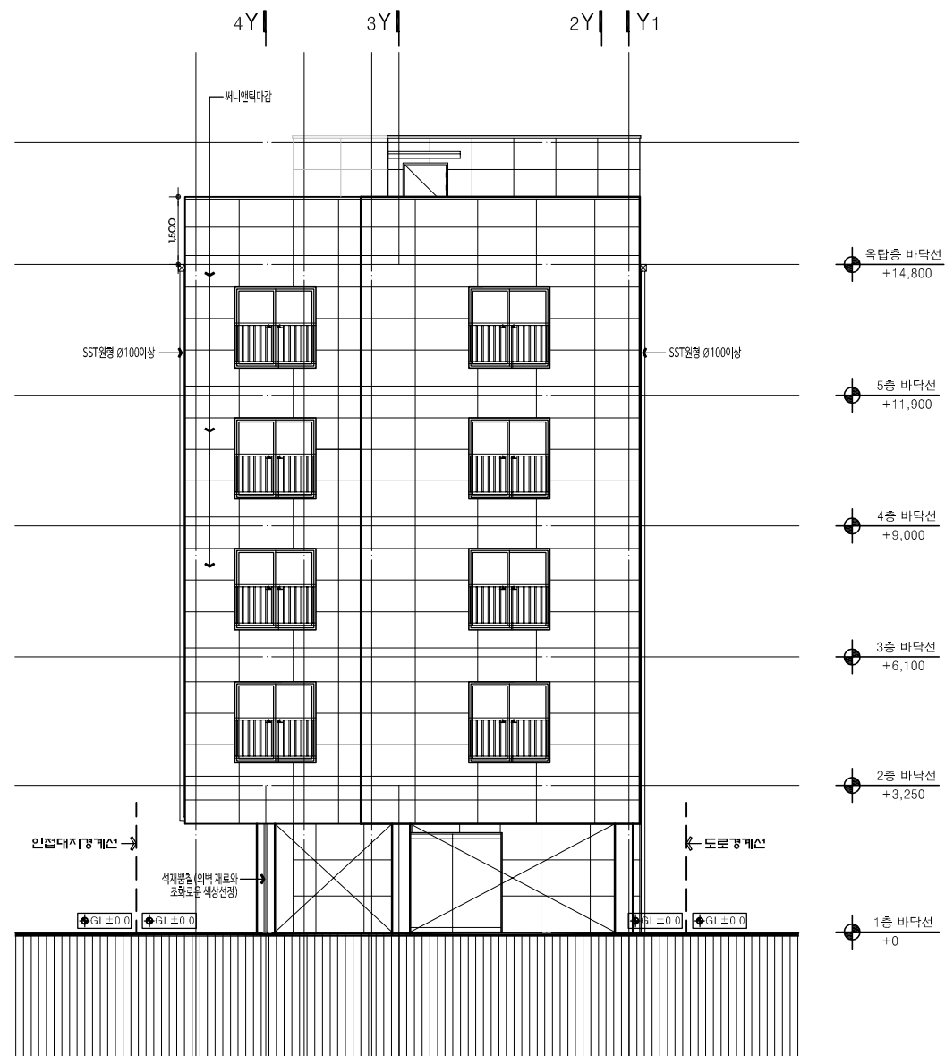
정면도 축척: 1/150
