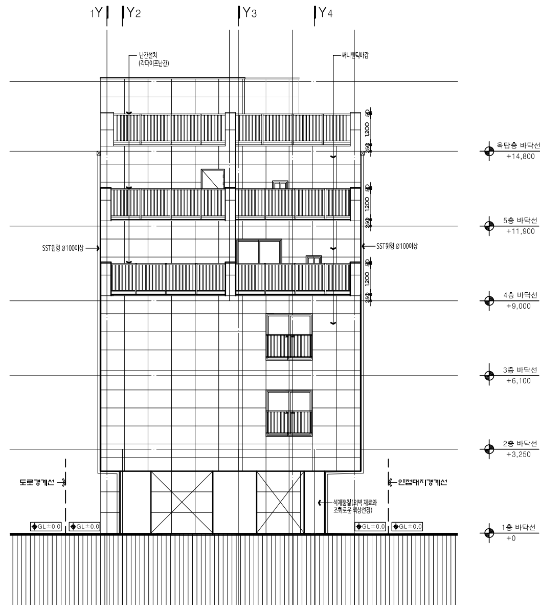
배 면 도 축척: 1/150
