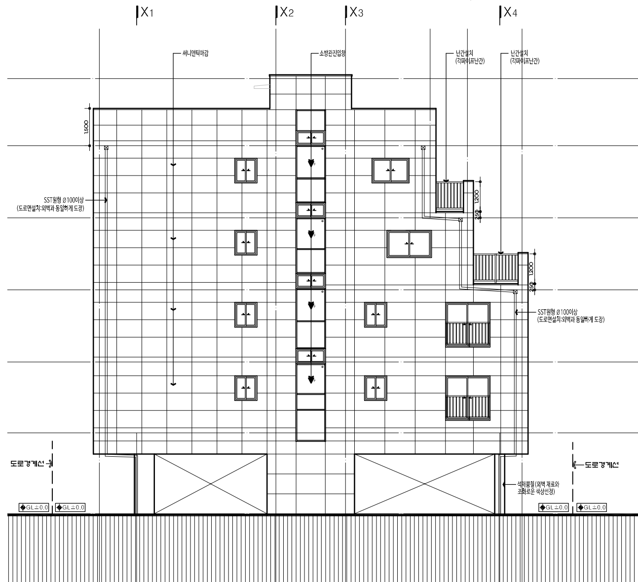
우측면도 축척: 1/150
