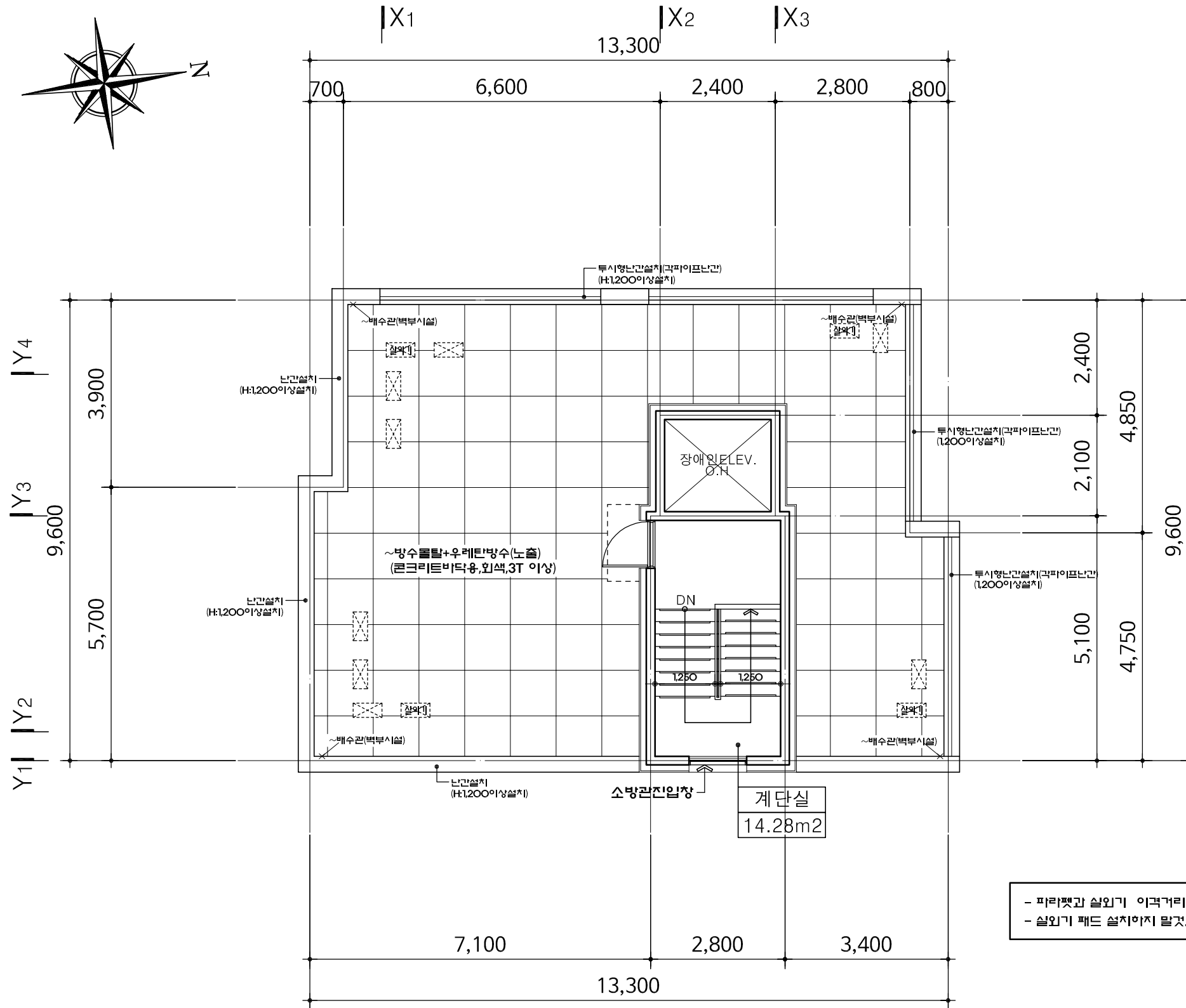
옥탑층 평면도 축척:1/100
